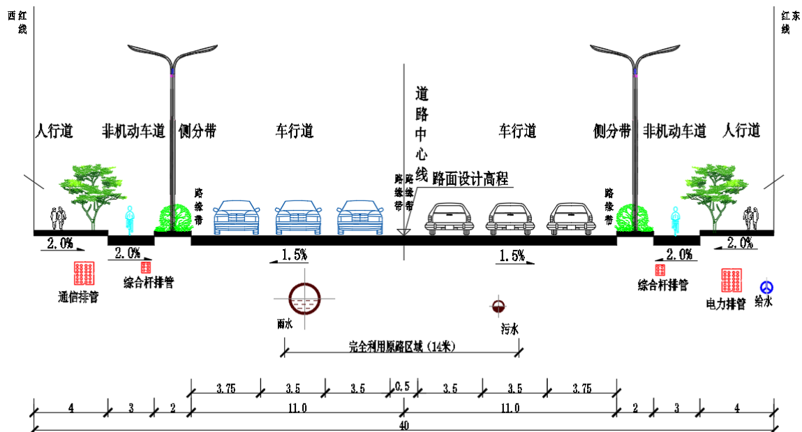
图 2.1-4 加宽段 K0+000-K0+622.025 标准横断面设计图
