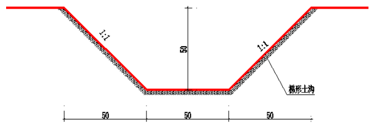
图 2.1-8 路基排水边沟断面设计图
