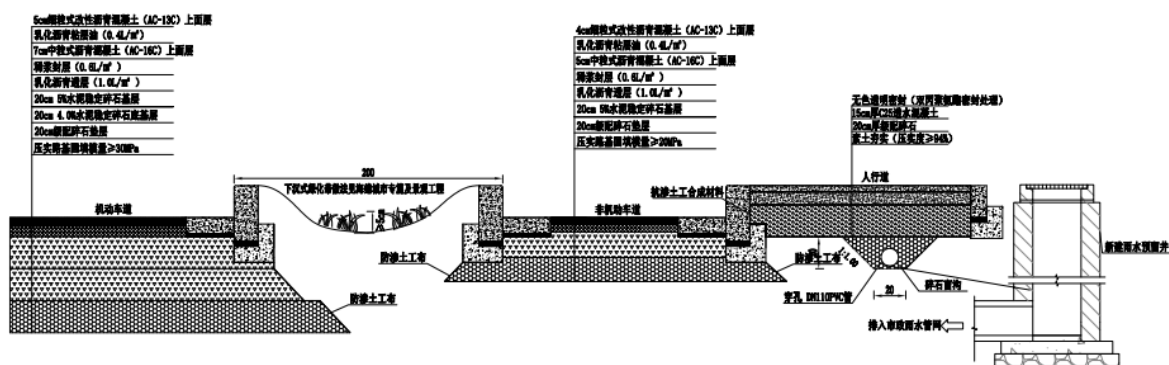
图 2.1-10 路面结构设计图
