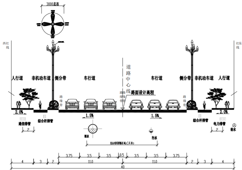
图 2.1-11 综合管线标准横断面图
