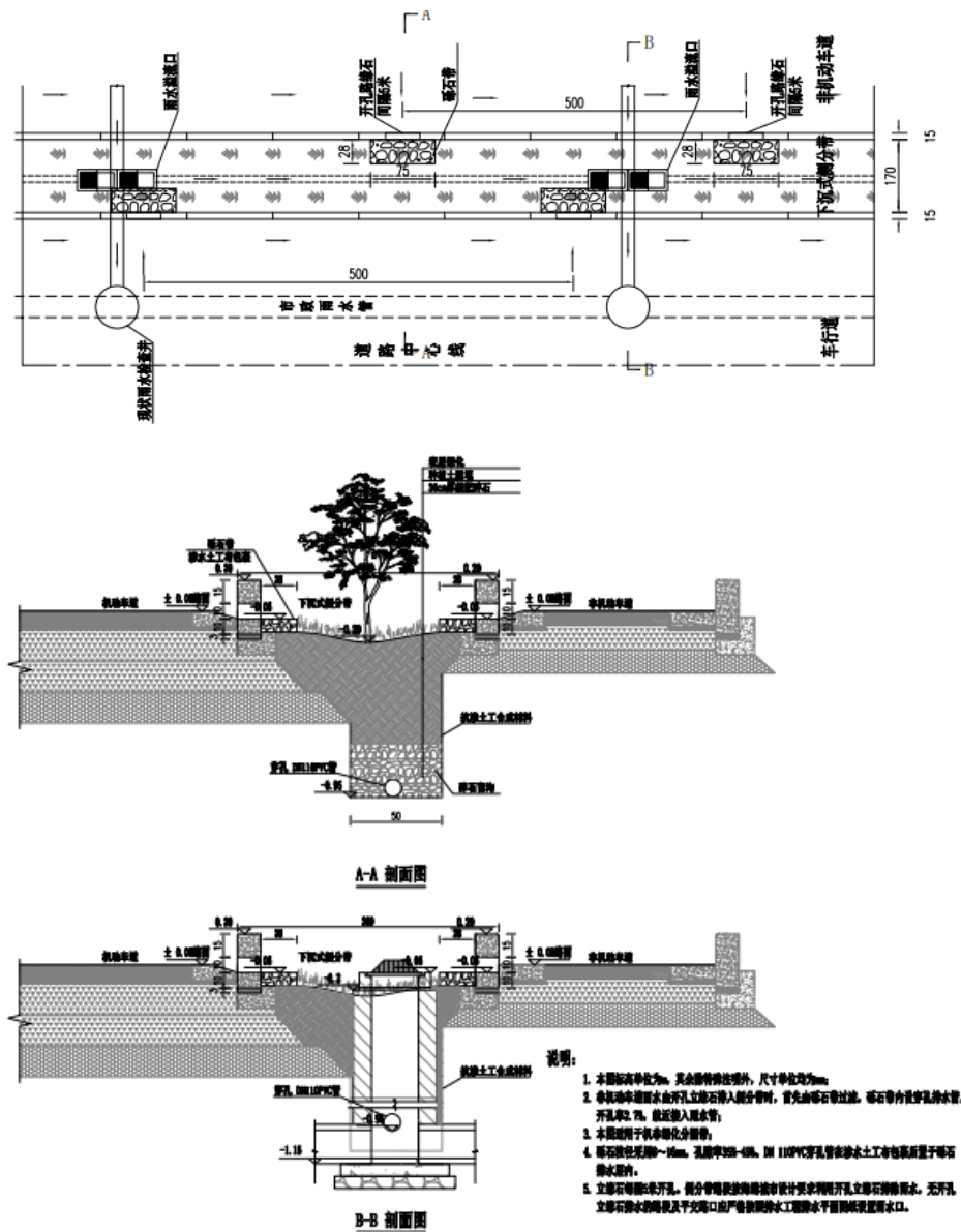
图 2.1-15 侧分带海绵设施布置图
