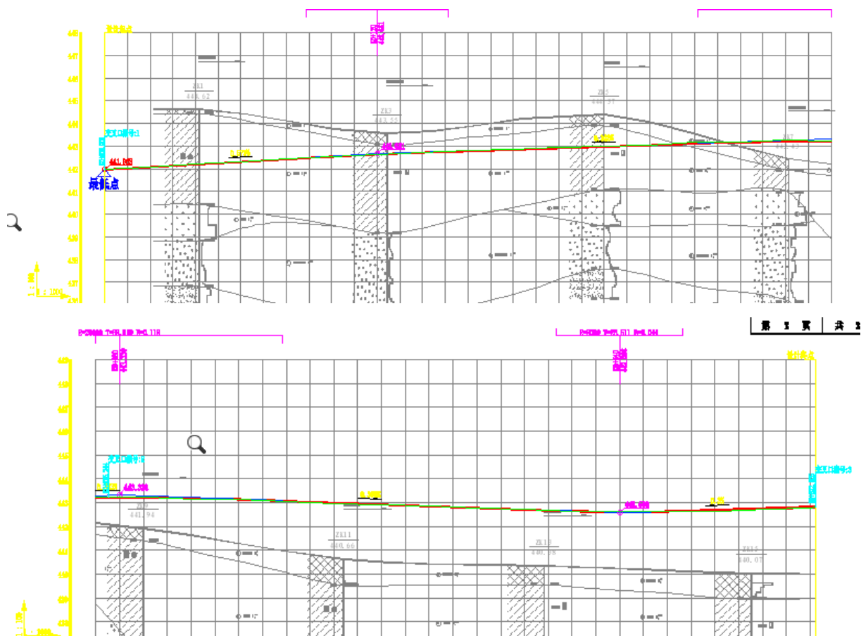
图 2.1-3 道路竖向布置图
