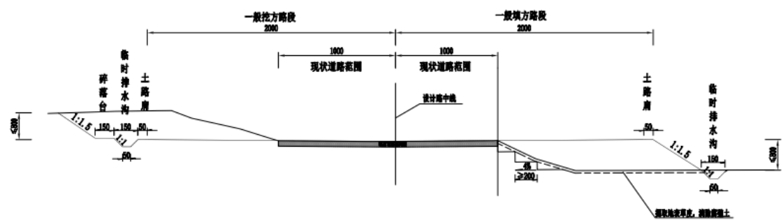
图 2.1-7 一般路基设计图
