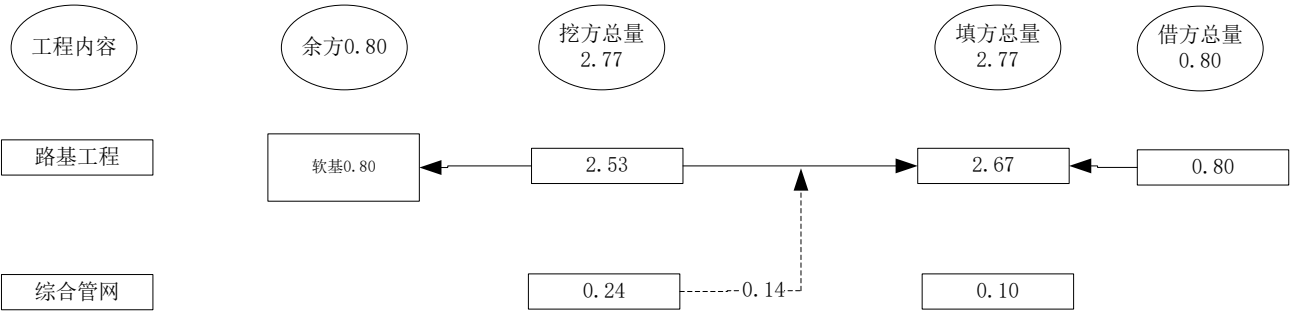
图 2.4-1 土石方流向框图
